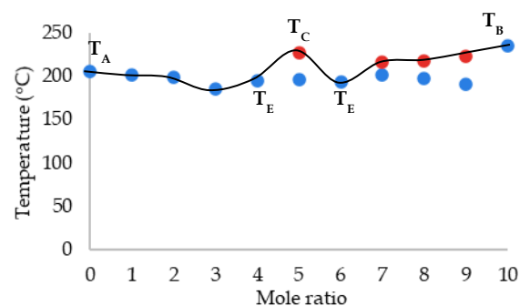
Figure 2. Phase diagram of GMP-MET binary systems. T_A : Melting point of GMP; T_B : Melting point of MET; T_C : Cocrystal point; T_E : Eutectic point. Mole ratio: 0 = GMP : MET (1 : 0); 1 = GMP : MET (9 : 1); 2 = GMP : MET (8 : 2); 3 = GMP : MET (7 : 3); 4 = GMP : MET (6 : 4); 5 = GMP : MET (5 : 5); 6 = GMP : MET (4 : 6); 7 = GMP : MET (3 : 7); 8 = GMP : MET (2 : 8); 9 = GMP : MET (1 : 9); 10 = GMP : MET (0 : 1)
