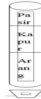
Gambar 1. Ilustrasi desain saringan pasir
